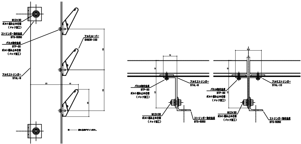
アルミルーバー SHGCW-100 アルミストリンガー STAL-9 STAL-10
