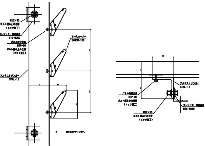
アルミルーバー SHGCW-100 アルミストリンガー STAL-11
