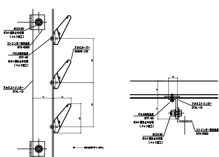
アルミルーバー SHGCW-100 アルミストリンガー STAL-13
