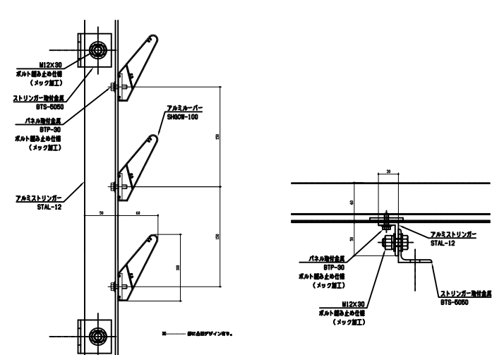
アルミルーバー SHGCW-100 アルミストリンガー STAL-12
