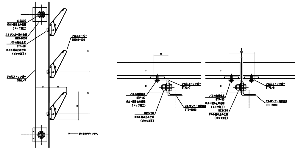
アルミルーバー SHGCW-100 アルミストリンガー STAL-8
