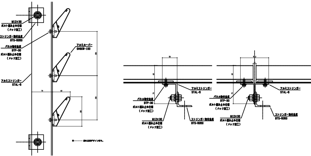
アルミルーバー SHGCW-100 アルミストリンガー STAL-5 STAL-6
