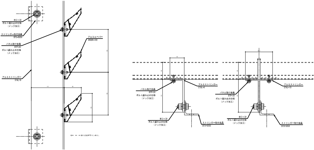
アルミルーバー SHGW-100 アルミストリンガー STAL-9 STAL-10
