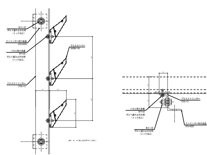
アルミルーバー SHGW-100 アルミストリンガー STAL-12
