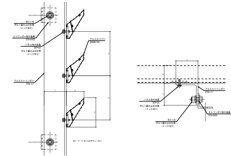
アルミルーバー SHGW-100 アルミストリンガー STAL-11
