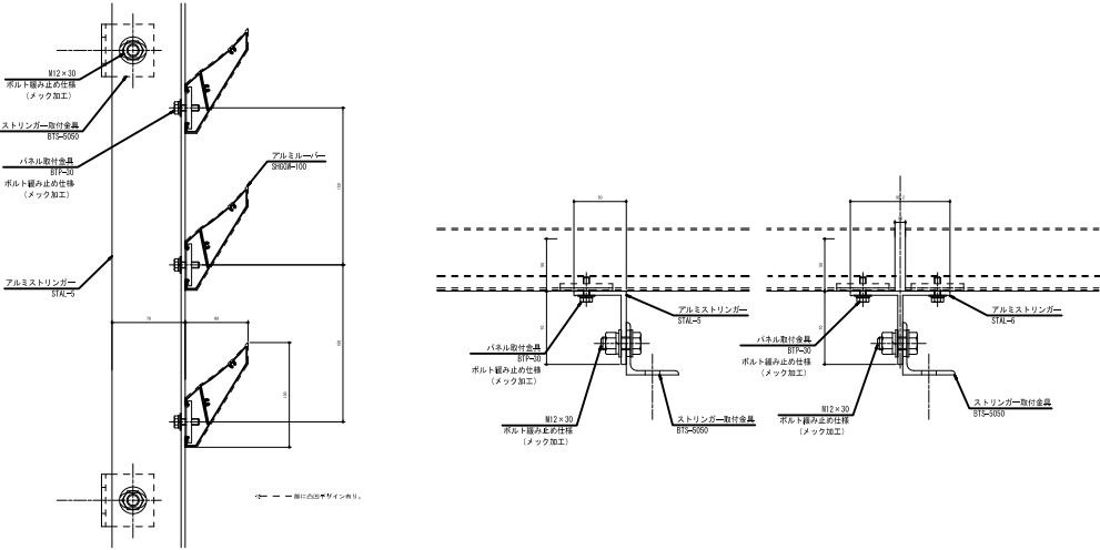
アルミルーバー SHGW-100 アルミストリンガー STAL-5 STAL-6
