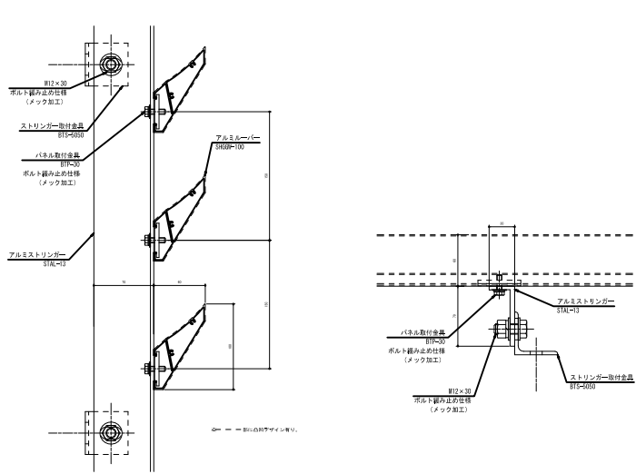
アルミルーバー SHGW-100 アルミストリンガー STAL-13
